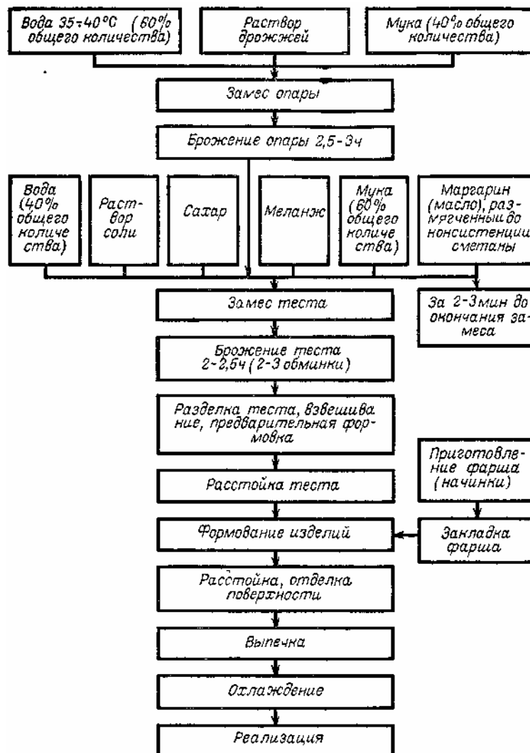
Рис 19 Технологическая схема изготовления изделий из дрожжевого теста, приготовленного опарным способом
