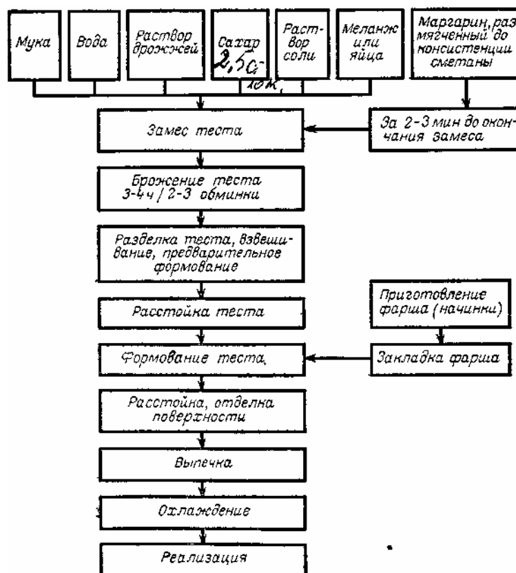
Рис. 18. Технологическая схема изготовления изделий из дрожжевого теста, приготовленного безопасным способом
